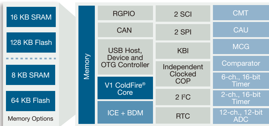
MCF51JM128顶层方框图
